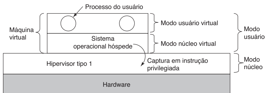
FIGURA 7.3 Quando o sistema operacional em uma máquina virtual executa uma instrução somente de núcleo, ele chaveia para o hipervisor com uma captura se a tecnologia de virtualização estiver presente.
