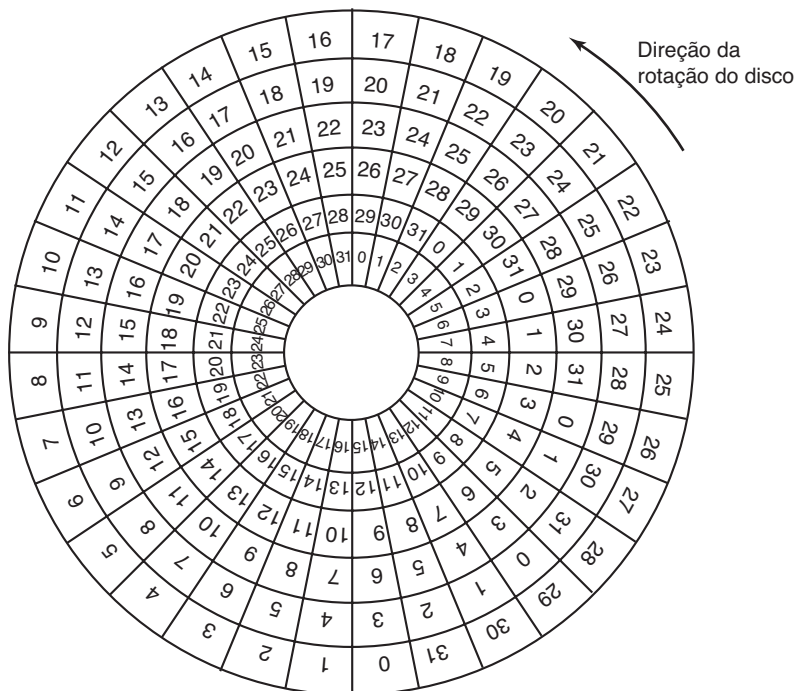
FIGURA 5.22 Uma ilustração do deslocamento de cilindro.
